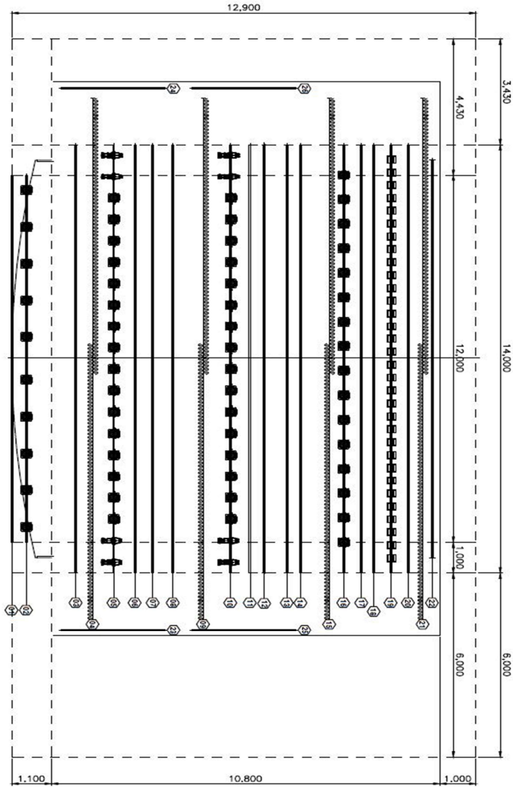
누림아트홀 상부기계배치도
